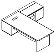
Model AZ01B(L/R) Size 2800(W)*2150(D)*750(H)mm 2400(W)*2150(D)*750(H)mm
