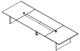
Model AH01 Size 4800(W)*1600(D)*750(H)mm
