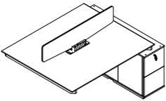
Model GY12 Size 1490(W)*1200(D)*750(H)mm 1690(W)*1200(D)*750(H)mm
