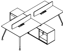
Model GY11 Size 1490(W)*1200(D)*750(H)mm 1690(W)*1200(D)*750(H)mm
